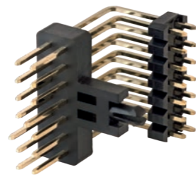
Sondersteckverbinder Sonderstiftleiste mit voreilenden Kontakten. Arretierung auf der Platinine
