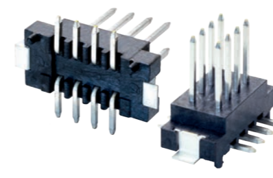
Stiftleiste mit Zentrierstiften Kundenspezifische Stiftleiste mit Zentrierstiften und zusätzlichen Löt pads
