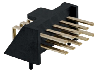
Sondersteckverbinder Sondersteckverbinder, abgewinkelt mit Ansaugfläche und verstärktem Isolierkörper
